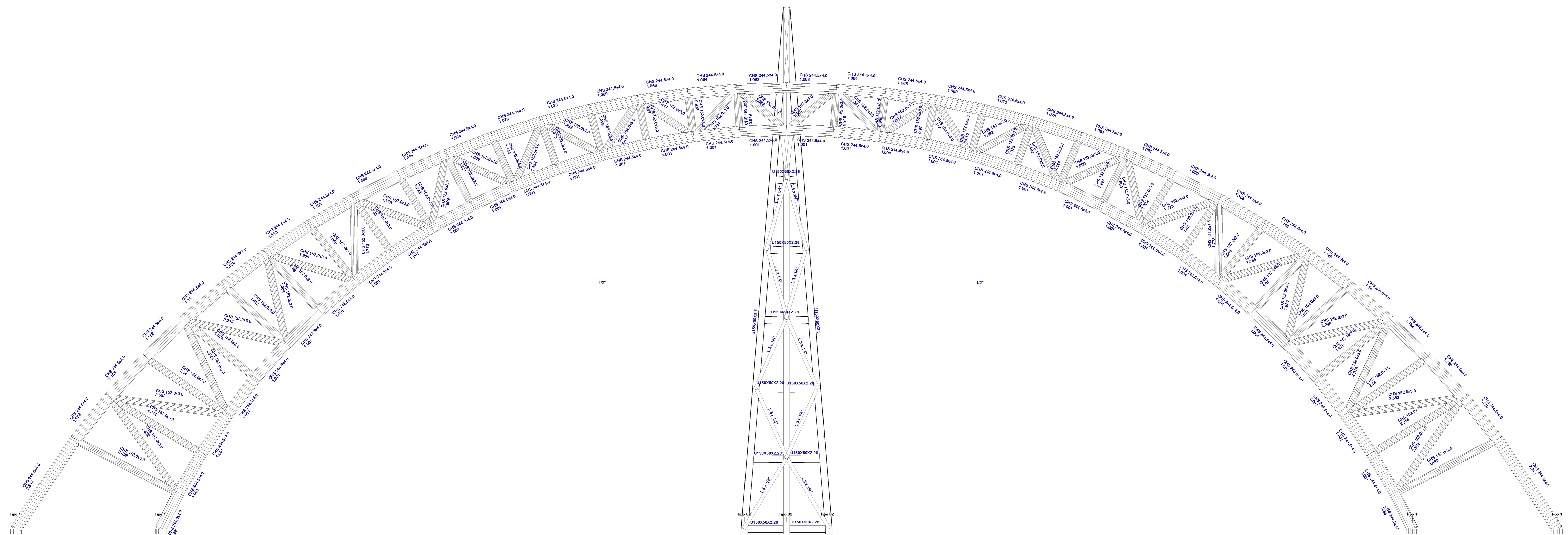
1 VISTA FRONTAL 1 : 30
