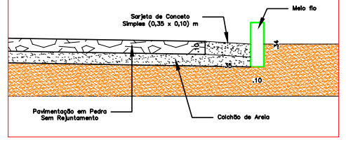
DETALHE DA SARJETA DE CONCRETO
