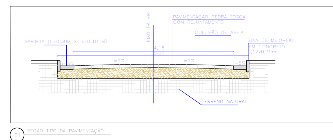
SEÇÃO TIPO DA PAVIMENTAÇÃO
