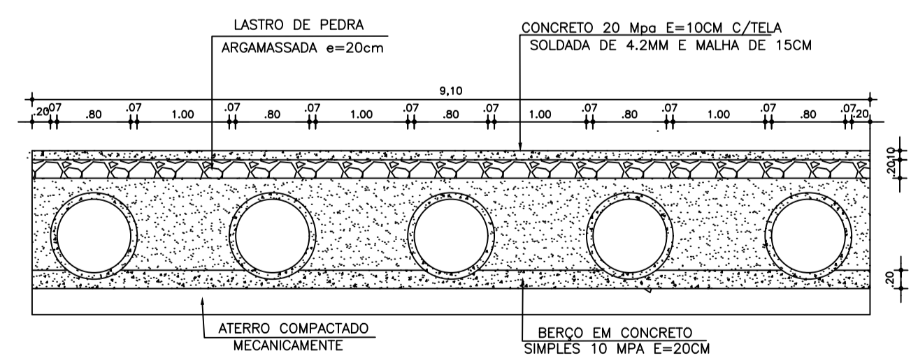
DETALHE DE COLOCAÇÃO DAS MANILHAS ESC.: 1/50
