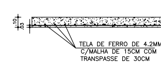
LAJE DA PISTA DE ROLAMENTO DETALHE DA COLOCAÇÃO DA TELA ESC.: 1/10
