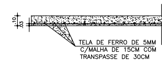
LAJE DA PISTA DE ROLAMENTO DETALHE DA COLOCAÇÃO DA TELA
