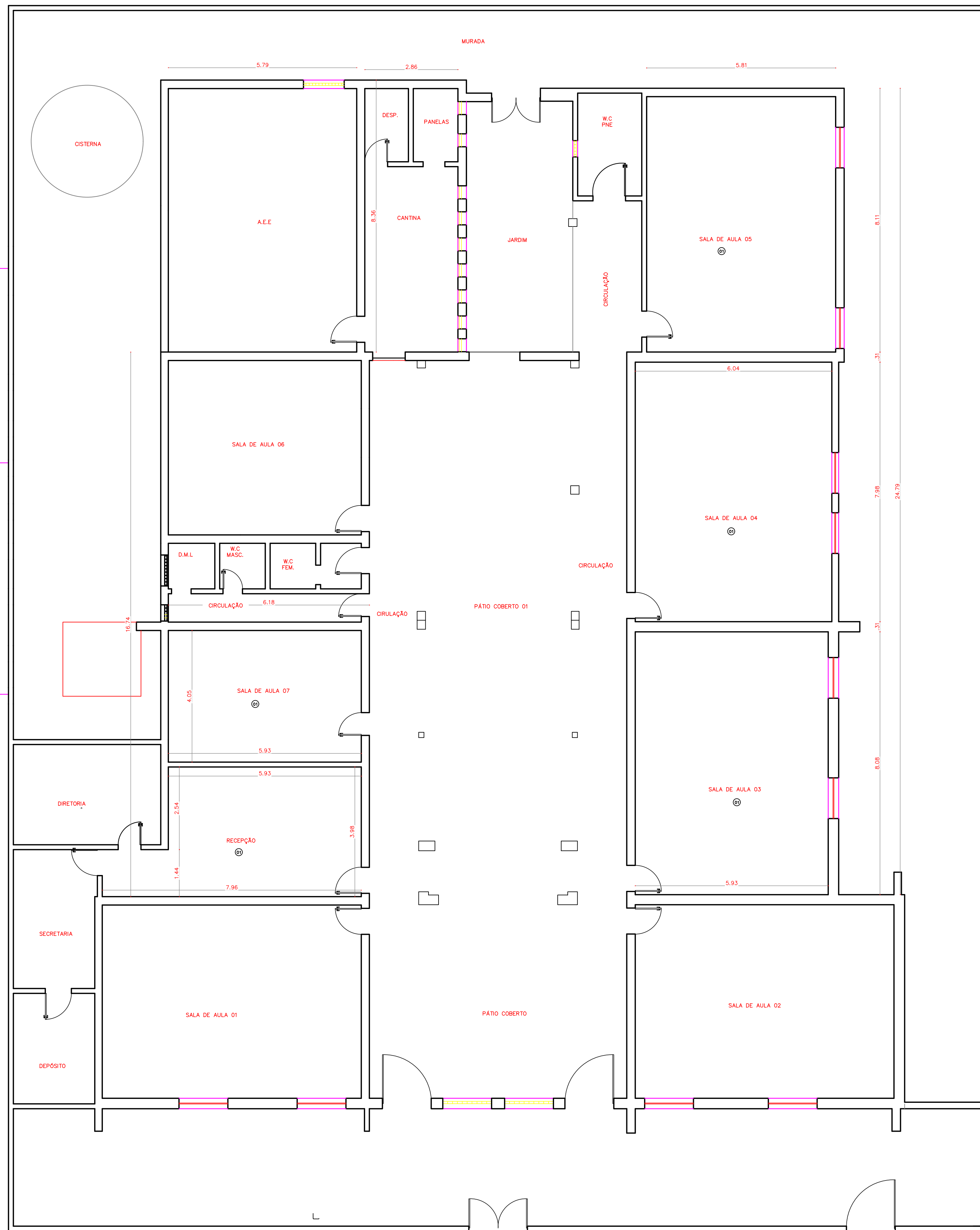
1. PLANTA BAIXA ATUAL Esc.: 1/75
