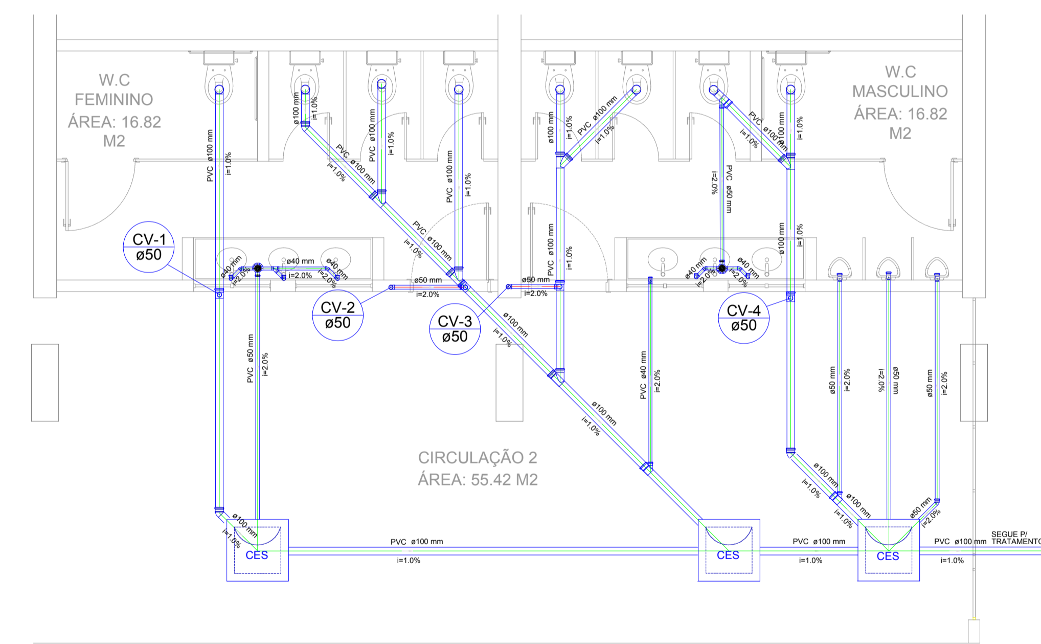
Detalhe S4 escala 1:50
