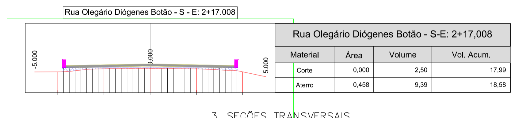
3. SEÇÕES TRANSVERSAIS Esc.: 1/100
