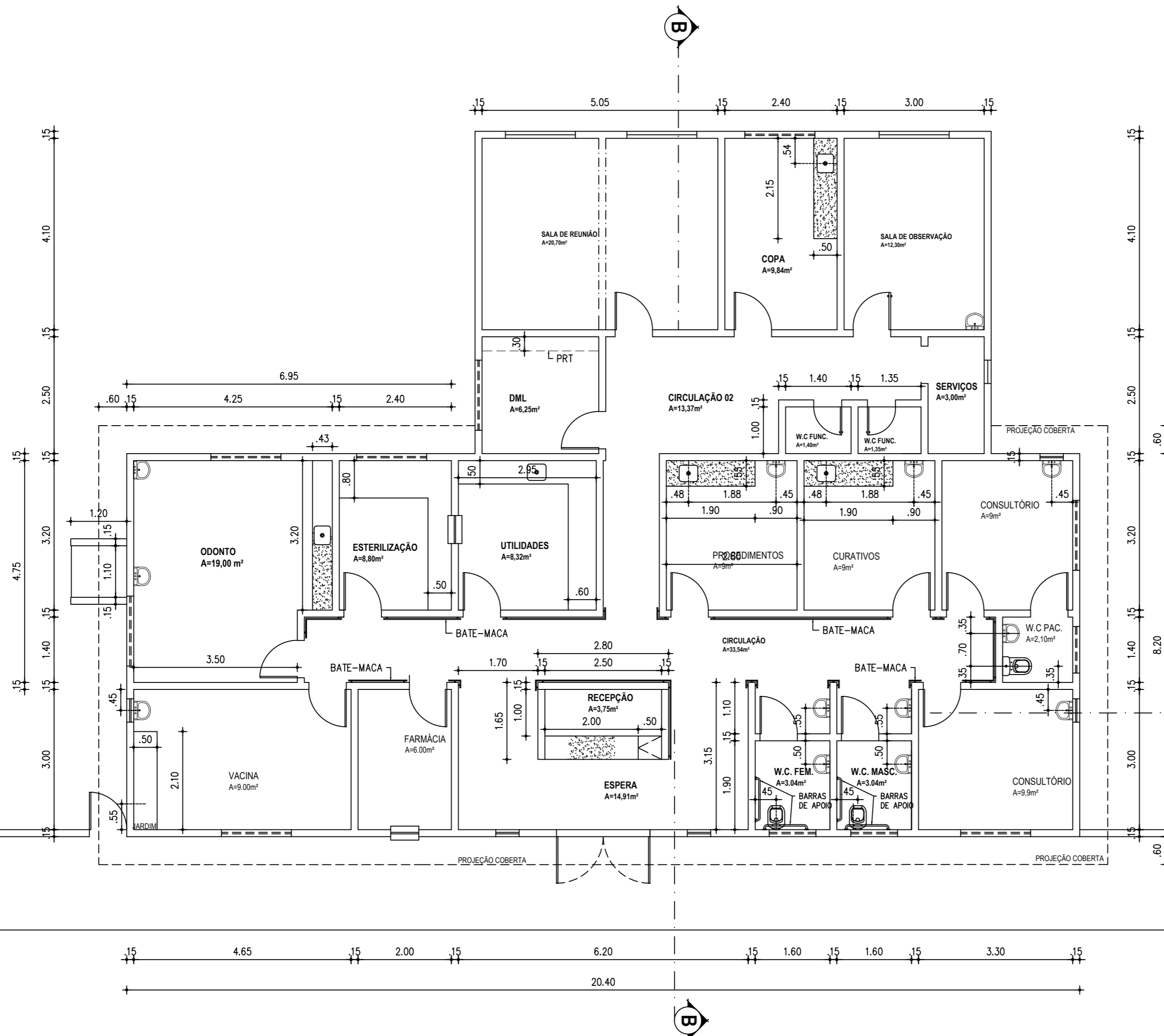
01 PLANTA BAIXA ESCALA: 1 / 75
