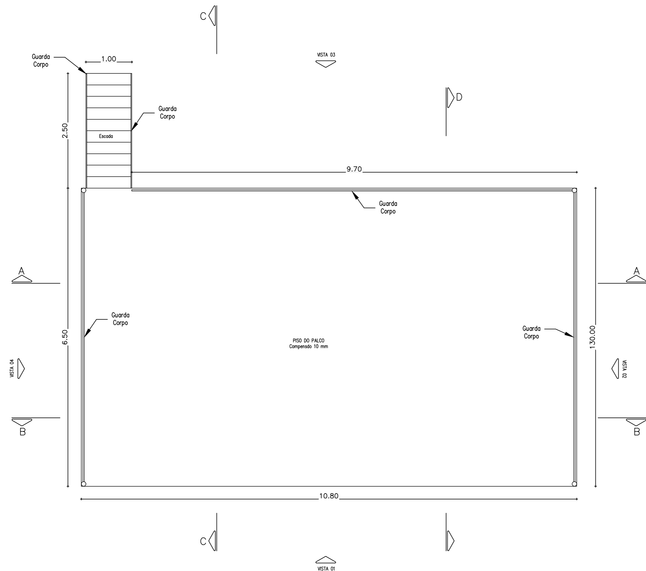
1. PLANTA BAIXA Esc.: 1/50
