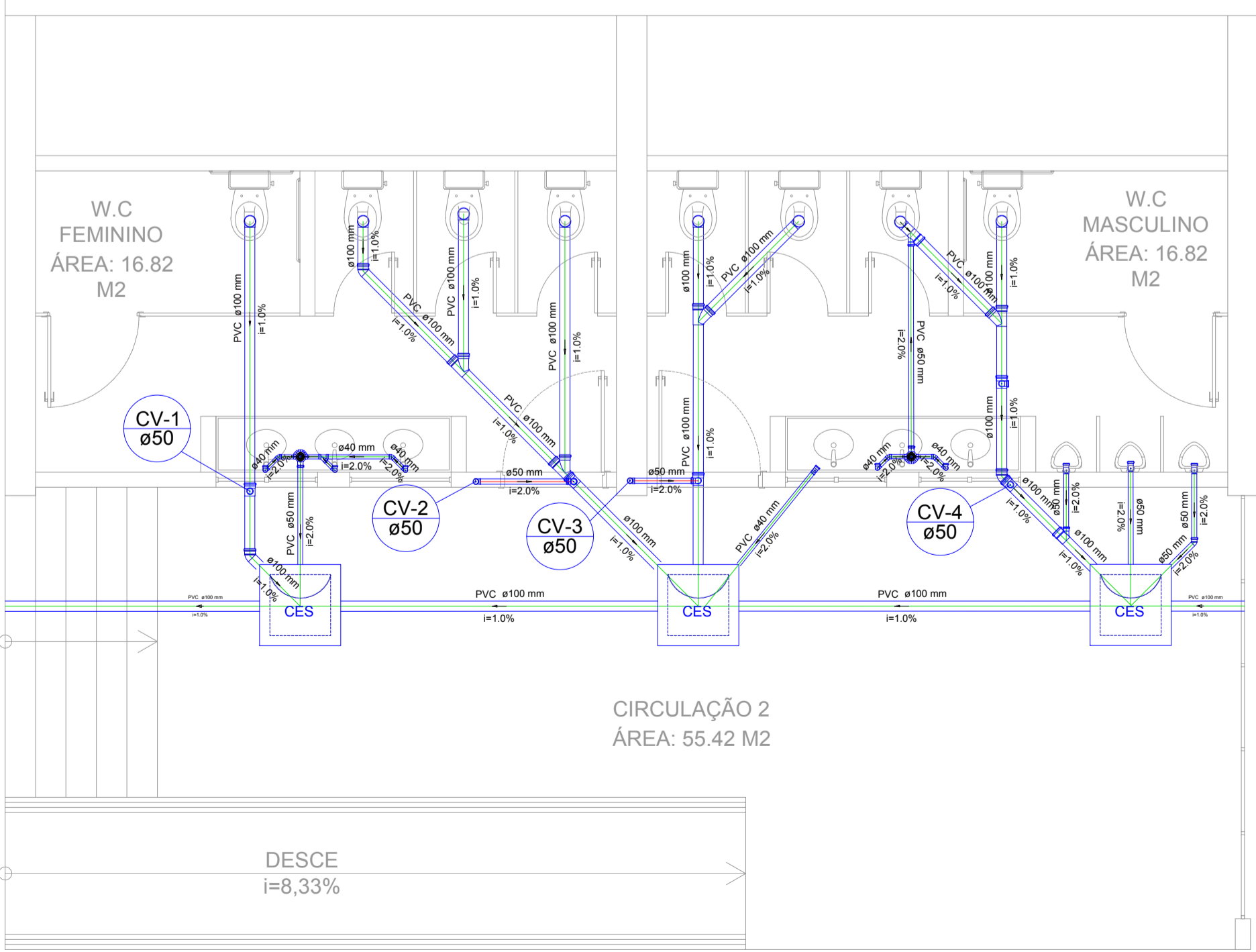
Detalhe S1 escala 1:50
