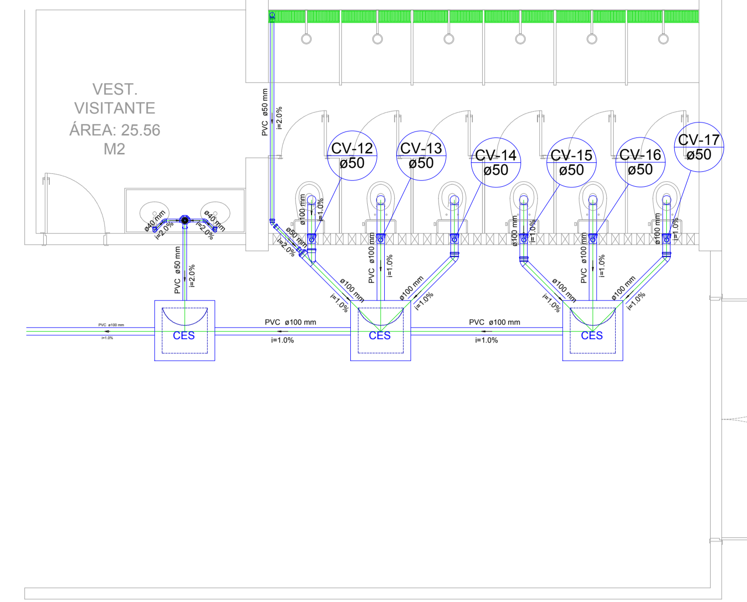
Detalhe S3 escala 1:50
