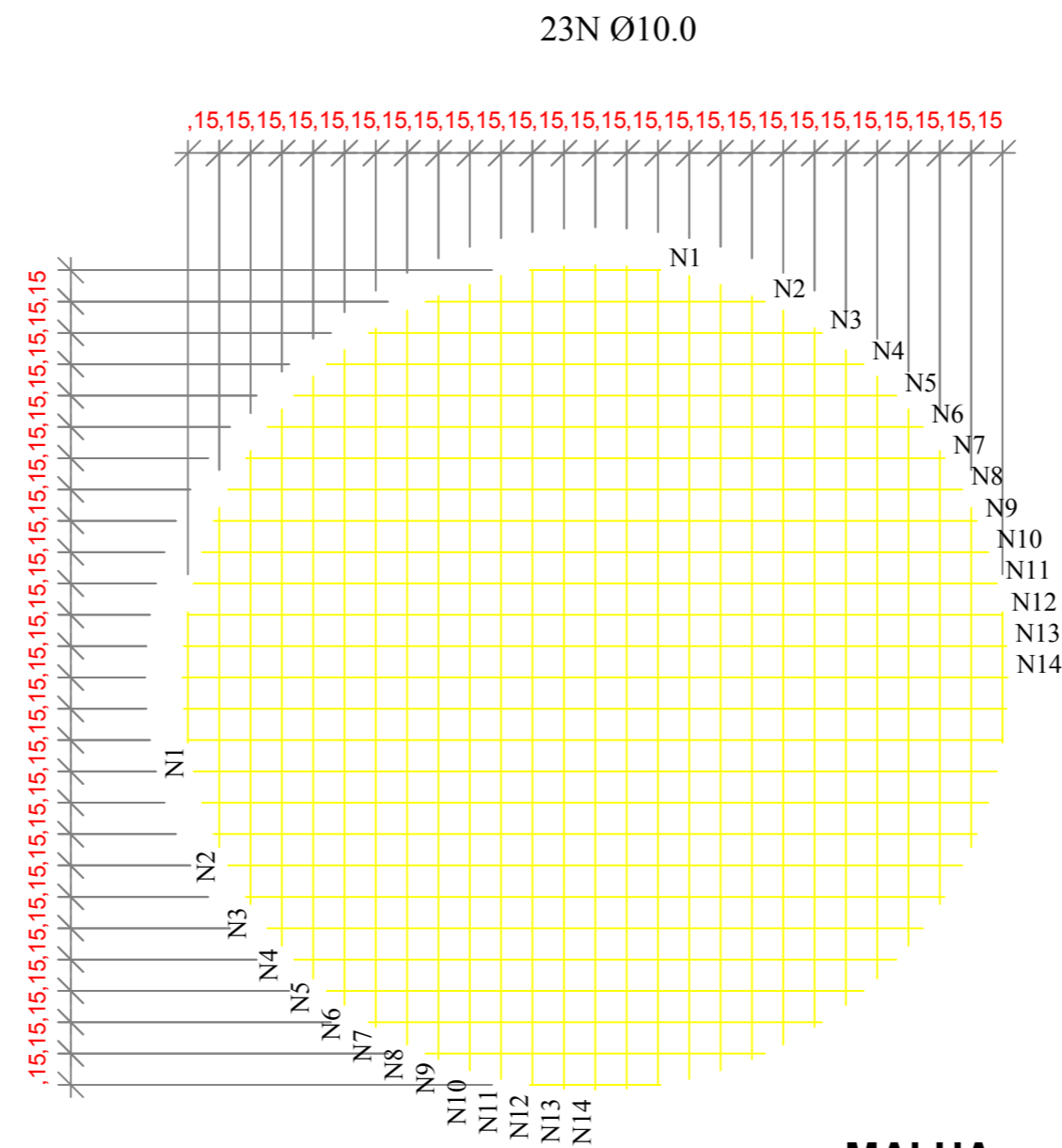
MALHA ESC. 1:50
