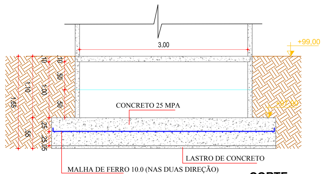
CORTE ESC. 1:50
