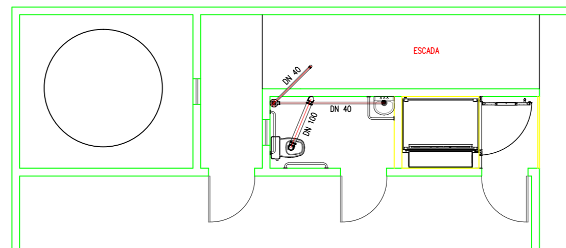
4. PLANTA BAIXA - SANITÁRIA SUPERIOR Esc.: 1/75
