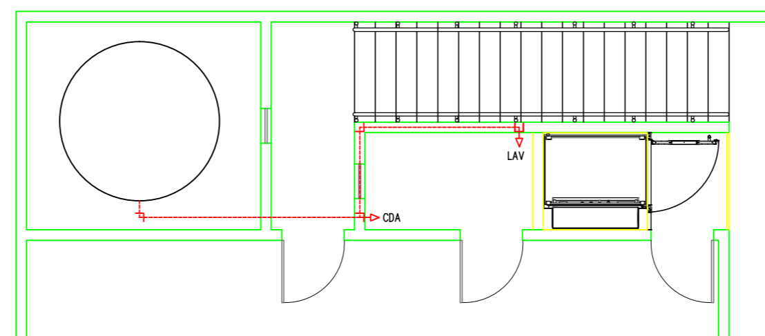
2. PLANTA BAIXA - HIDRÁULICA SUPERIOR Esc.: 1/75
