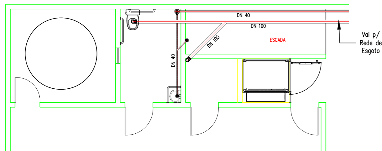
3. PLANTA BAIXA - SANITÁRIA TÉRREO Esc.: 1/75
