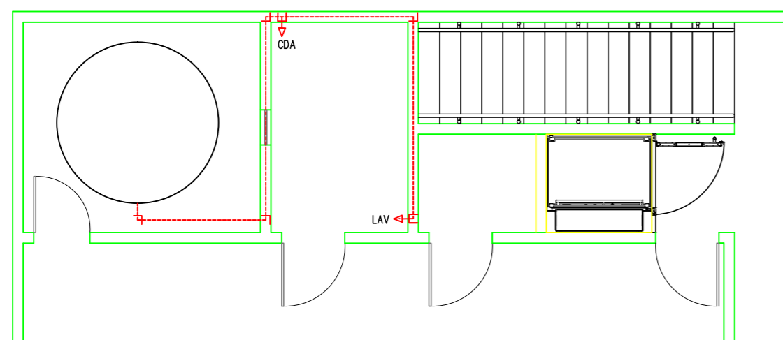
1. PLANTA BAIXA - HIDRÁULICA TÉRREO Esc.: 1/75
