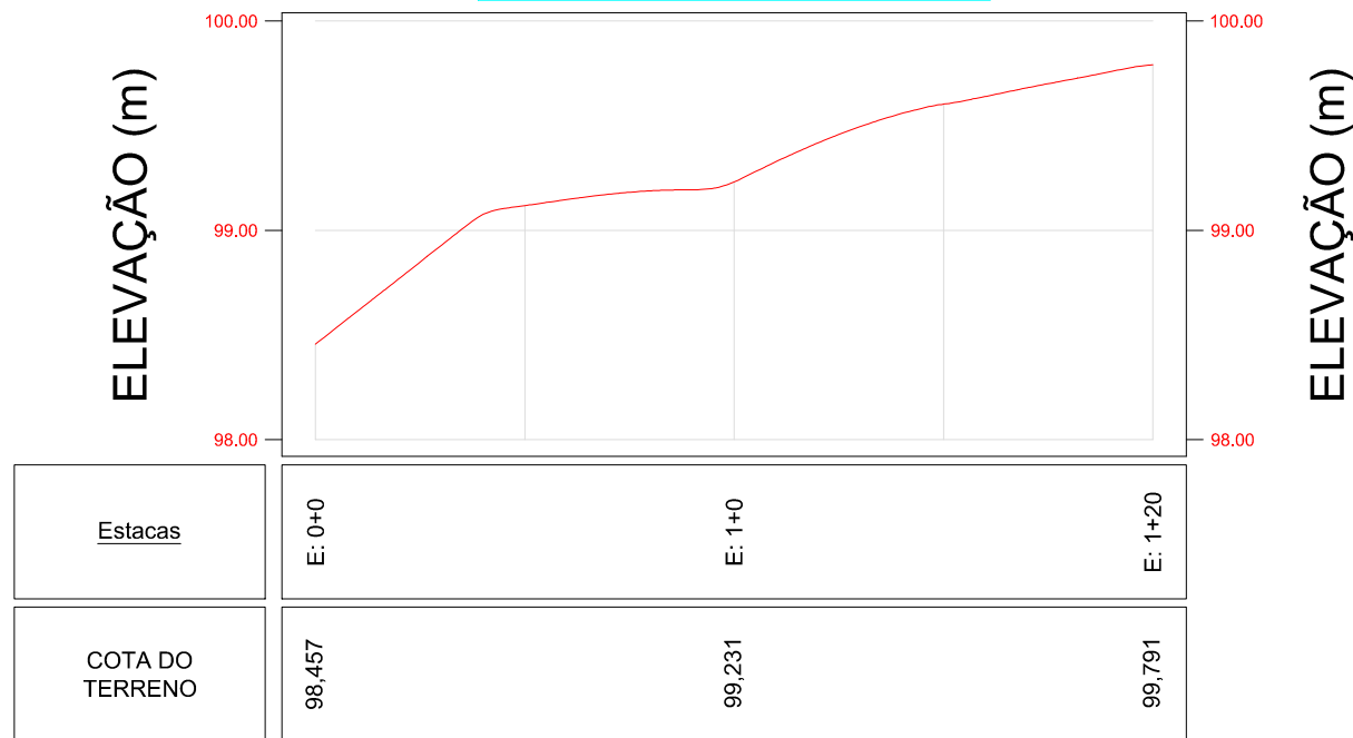
PERFIL - TERRENO 01 (Escala Vertical: 25)
