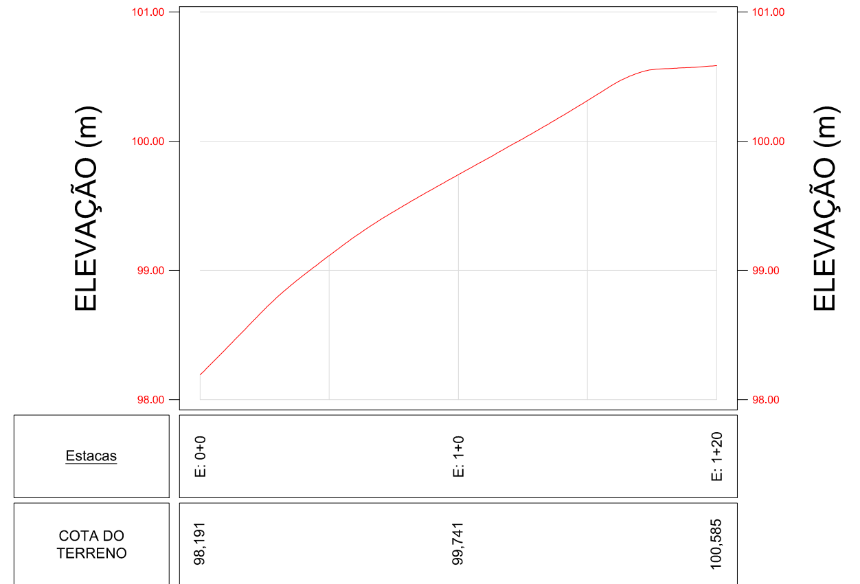
PERFIL - TERRENO 02 (Escala Vertical: 25)
