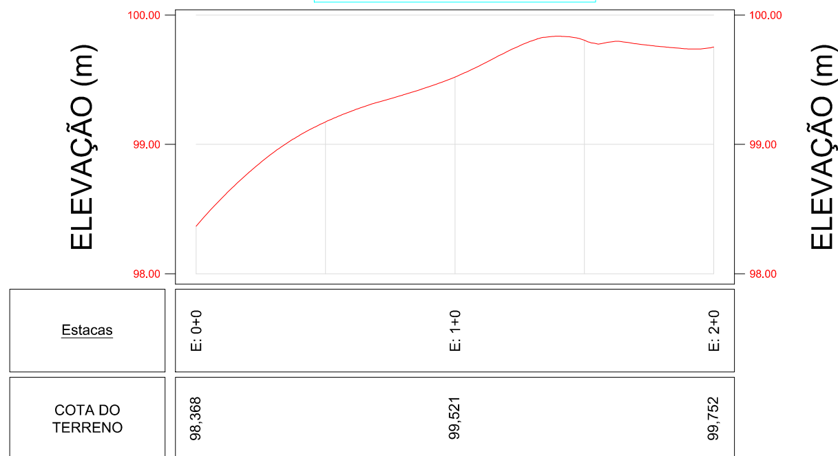
PERFIL - TERRENO (Escala Vertical: 25)
