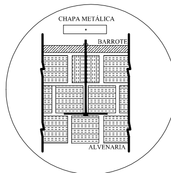
DETALHE DE AMARRAÇÃO DO BARROTE
