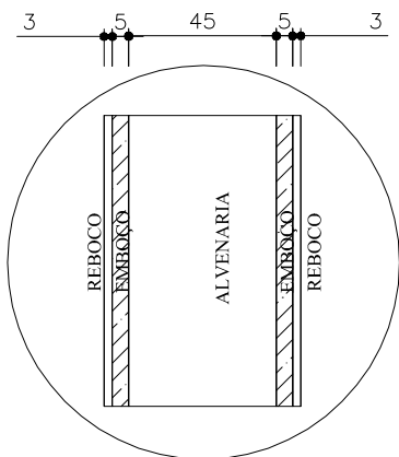
DETALHE DO REVESTIMENTO DA PAREDES ESC. : 1:5
