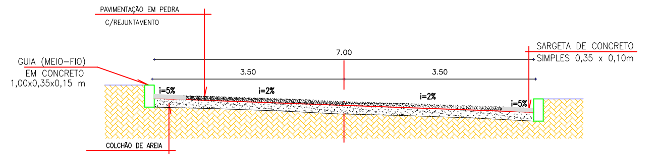
2. SEÇÃO TIPO Esc.: Sem Escala
