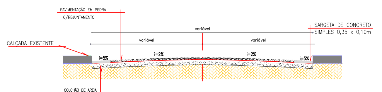
3 . SEÇÃO TIPO 02 Esc.: Sem Escala
