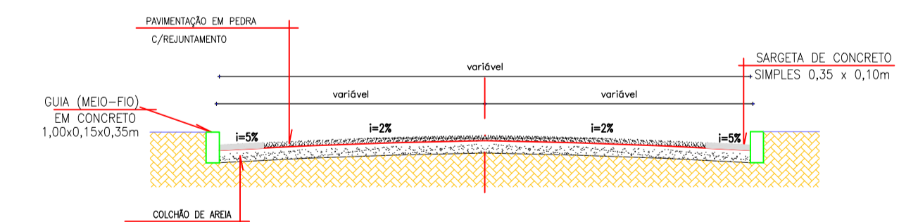
2 . SEÇÃO TIPO 01 Esc.: Sem Escala
